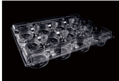
型号: JM-119 十二枚糕点盒 装箱: 100个 材质: PET 尺寸: (外) 390mm*295mm*70mm 单粒最大尺寸: Ø85mm*68mm
