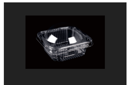
型号: JM-7028 装箱: 2000个 材质: PET 尺寸: (外) 73mm*73mm*50mm (内) 60mm*60mm*48mm
