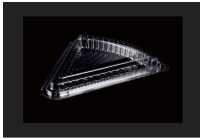
型号: JM-030三角披萨盒 装箱: 400个 材质: PET 尺寸: (外) 217mm*210mm*35mm (内) 193mm*180mm*33mm
