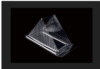
型号: JM-012 装箱: 2100个 材质: PET 尺寸: (外) 165mm*85mm*90mm (内) 144mm*75mm*80mm
