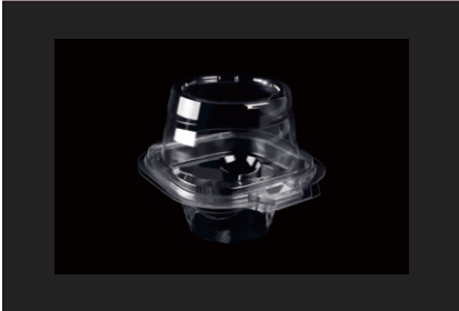
型号: JM-094马芬单格 装箱: 600个 材质: PET 尺寸: (外) 110mm*100mm*90mm (内) 80mm*80mm*88mm
