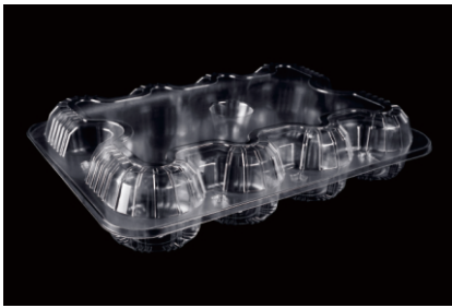
型号: JM-083 十枚烧麦盒 装箱: 200个 材质: BOPS 尺寸: (外) 275mm*195mm*55mm 单粒最大直径: Ø63mm
