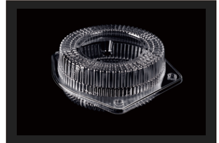
型号: JM-098 装箱: 600个 材质: PET 尺寸: (外) 175mm*170mm*65mm (内) 157mm*157mm*63mm
