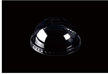
型号: JM-98G 装箱: 1000个 材质: PET 尺寸: Ø98mm*44mm
