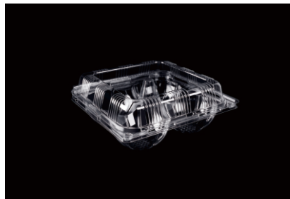
型号: JM-S04A小四枚果盒 装箱: 400个 材质: PET 尺寸: (外) 192mm*192mm*80mm 单粒最大直径: Ø78mm
