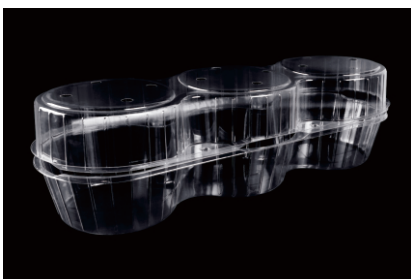
型号: JM-3X三个西兰花盒 装箱: 100个 材质: PET 尺寸 (外) 430mm*150mm*120mm 单粒最大直径: Ø135mm
