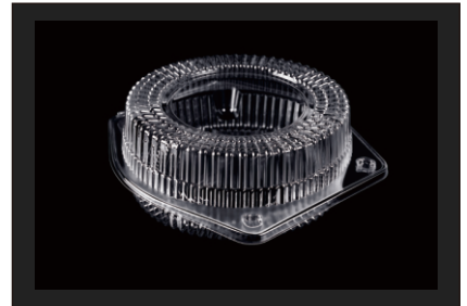
型号: JM-098 装箱: 600个 材质: PET 尺寸: (外) 175mm*170mm*65mm (内) 157mm*157mm*63mm
