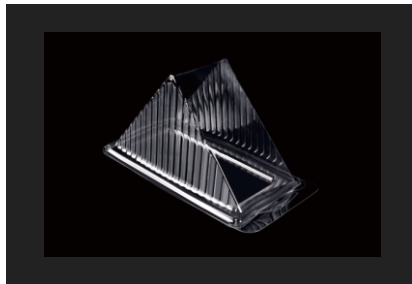
型号: JM-012 装箱: 2100个 材质: PET 尺寸: (外) 165mm*85mm*90mm (内) 144mm*75mm*80mm
