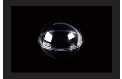
型号: JM-092椰子蛋盒 装箱: 400个 材质: PET 尺寸: (外) Ø130mm*120mm (内) Ø120mm*118mm
