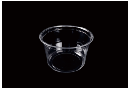
型号: JM-117-16oz 装箱: 500个 材质: PET 尺寸: Ø117mm*76mm 容量: 约550ml
