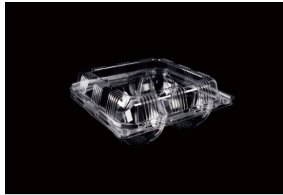
型号: JM-S04A小四枚果盒 装箱: 400个 材质: PET 尺寸: (外) 192mm*192mm*80mm 单粒最大直径: Ø78mm
