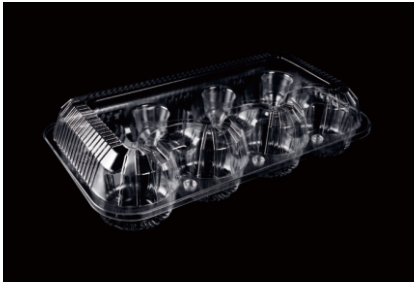
型号: JM-053 八枚烧麦盒 装箱: 300个 材质: BOPS 尺寸: (外) 260mm*145mm*63mm 单粒最大直径: Ø60mm
