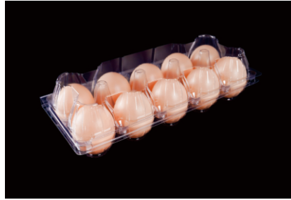
型号: JM-D10 大号鸡蛋托 装箱: 560个 材质: PET 尺寸: (外) 250mm*105mm*75mm 单粒最大直径: Ø45mm
