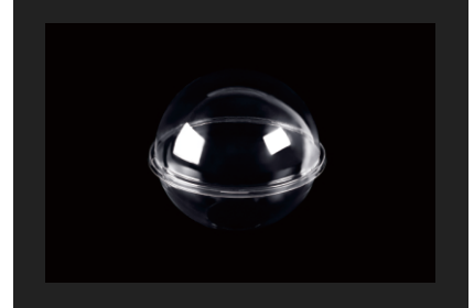
型号: JM-092椰子蛋盒 装箱: 400个 材质: PET 尺寸: (外) \varnothing 130mm*120mm (内) \varnothing 120mm*118mm
