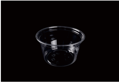
型号: JM-117-14oz 装箱: 500个 材质: PET 尺寸: Ø117mm*69mm 容量: 约450ml
